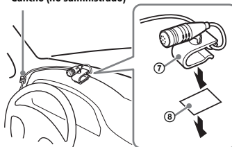
Gancho (no suministrado)
