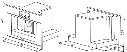
Product wordt op rails in de nis geplaatst: de rails zijn 450 mm lang
