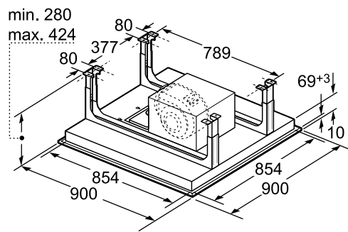
Afmetingen in mm
