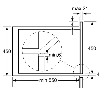
Afmetingen in mm
