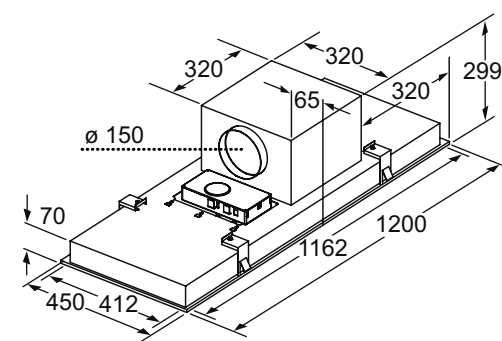
Afmetingen in mm
