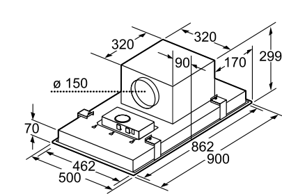
Afmetingen in mm
