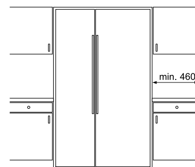
Afmetingen in mm
