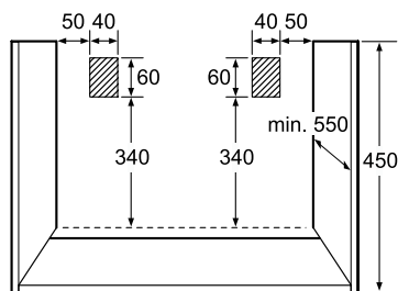
Afmetingen in mm
