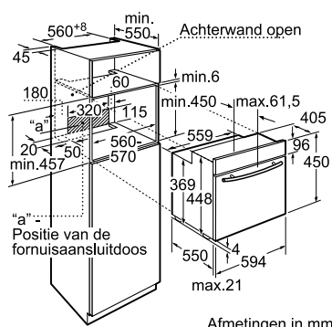
Afmetingen in mm
