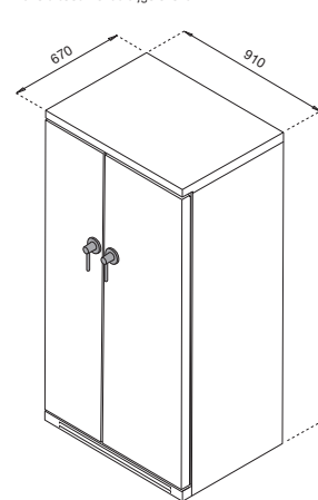
Buitenmaat geïntegreerd
