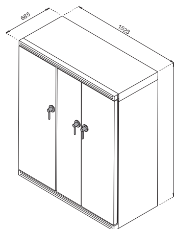
Buitenmaat geïntegreerd
