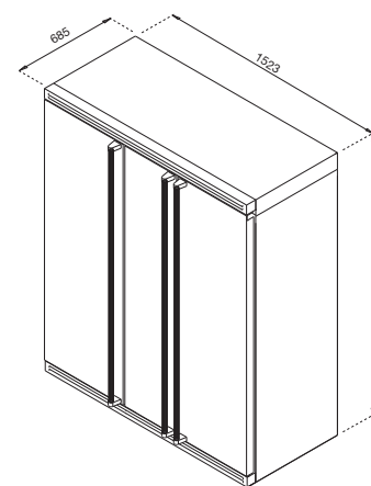
Inbouwmaat geïntegreerd
