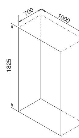
Inbouwmaat geïntegreerd
