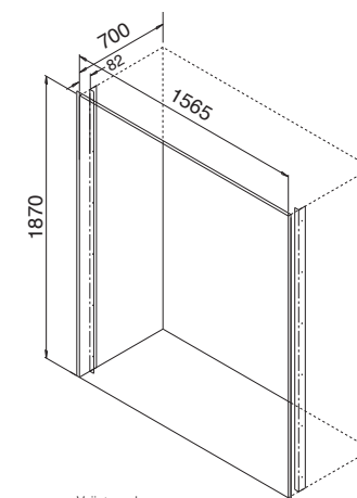
Vrijstaand
