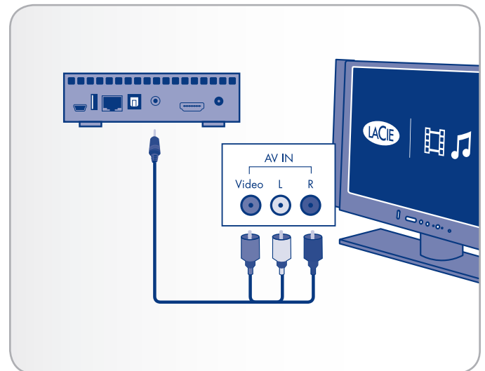
Afb. 24 - Samengestelde aansluiting
