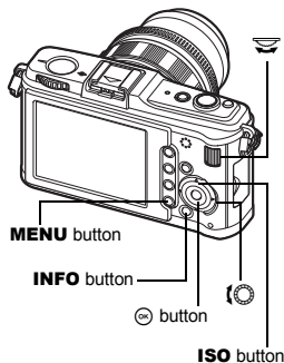
ISO button
