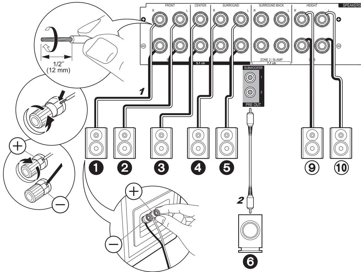
1 Lautsprecherkabel, 2 Subwoofer-Kabel
