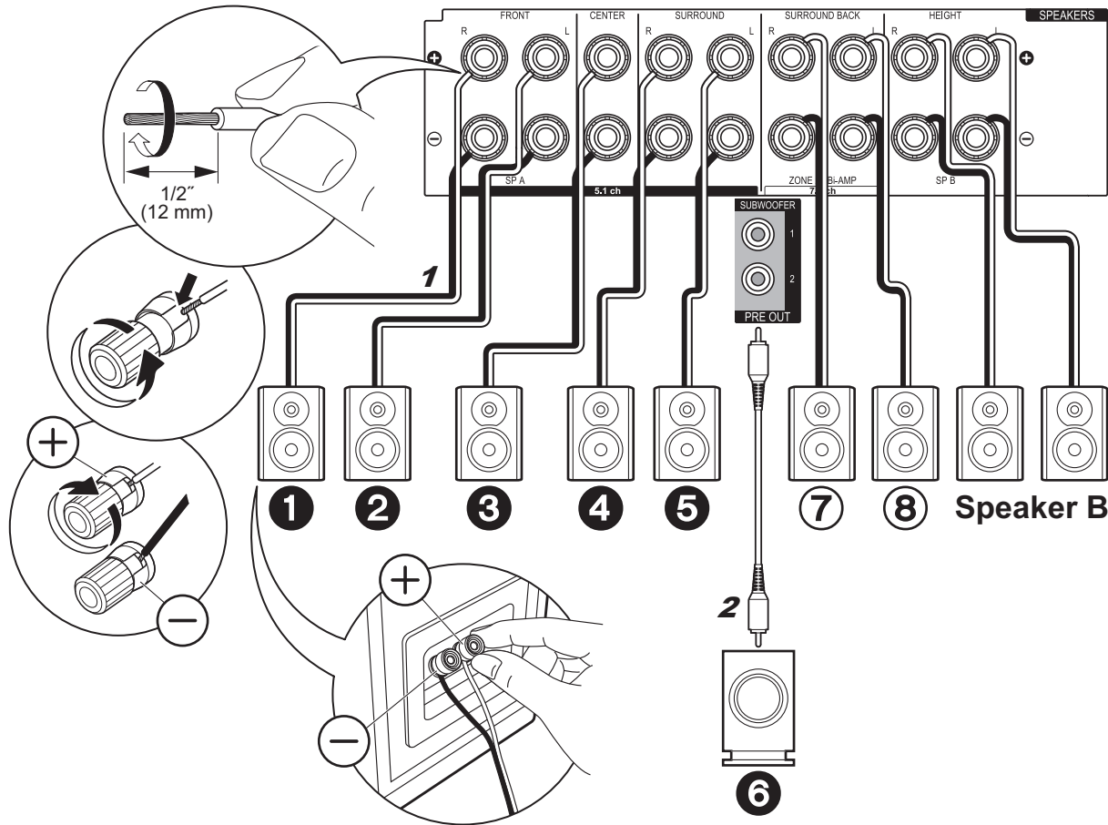
1 Lautsprecherkabel, 2 Subwoofer-Kabel
