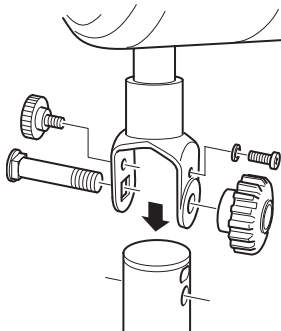
Abbildung 4 Den Ventilator auf dem Stativ anbringen
