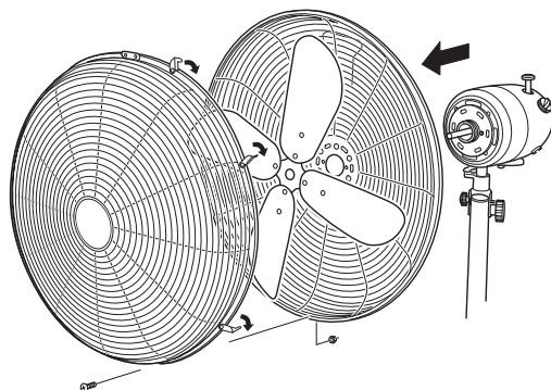
Figura 8 esensamble completamente las partes antes de hacer la limpieza o el mantenimiento
