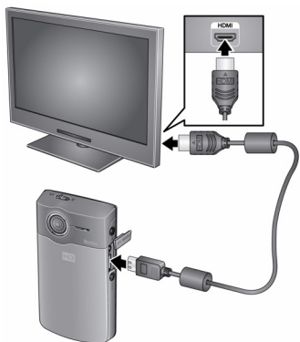
HDMI-kabel
