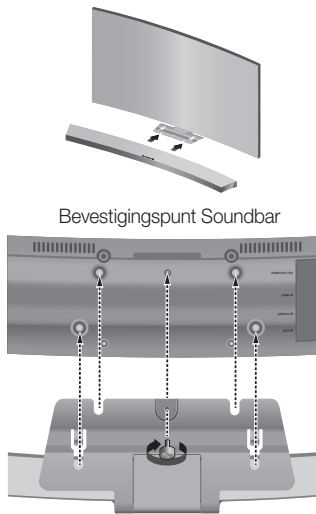
Tv-voet met bevestigde Montage-Beugel
